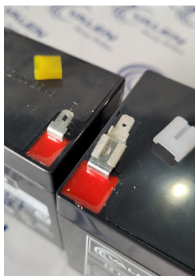
Convert F2 Battery Terminals to F1
